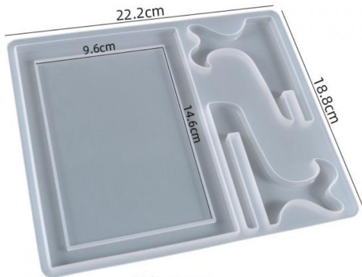
厚度: 0.9cm 成品尺寸: 12.4*17.4*0.8cm 长方相框架模具
