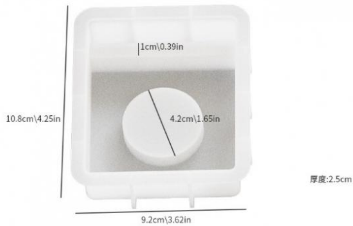
正方单孔底座004
