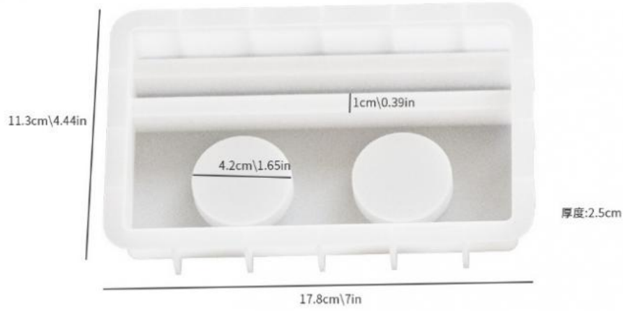
长方双孔底座001
