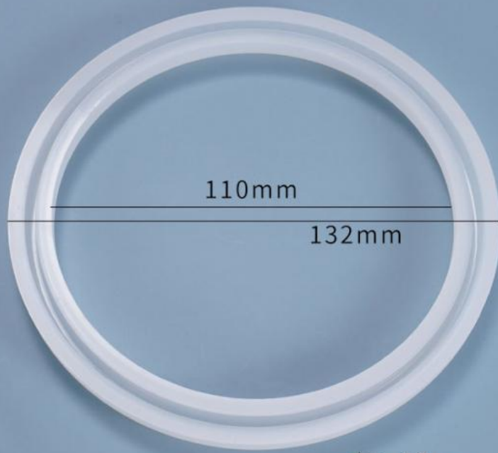
高：12mm 成品内径：110mm 圆环110硅胶模具
