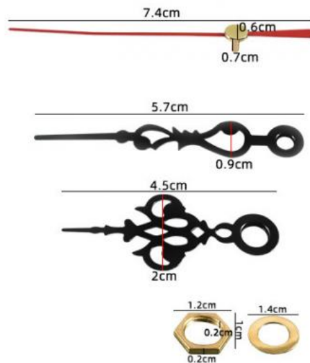
钟表芯-指针 (黑色)
